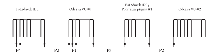
Obrázek 1 Tok zprávy, časování
