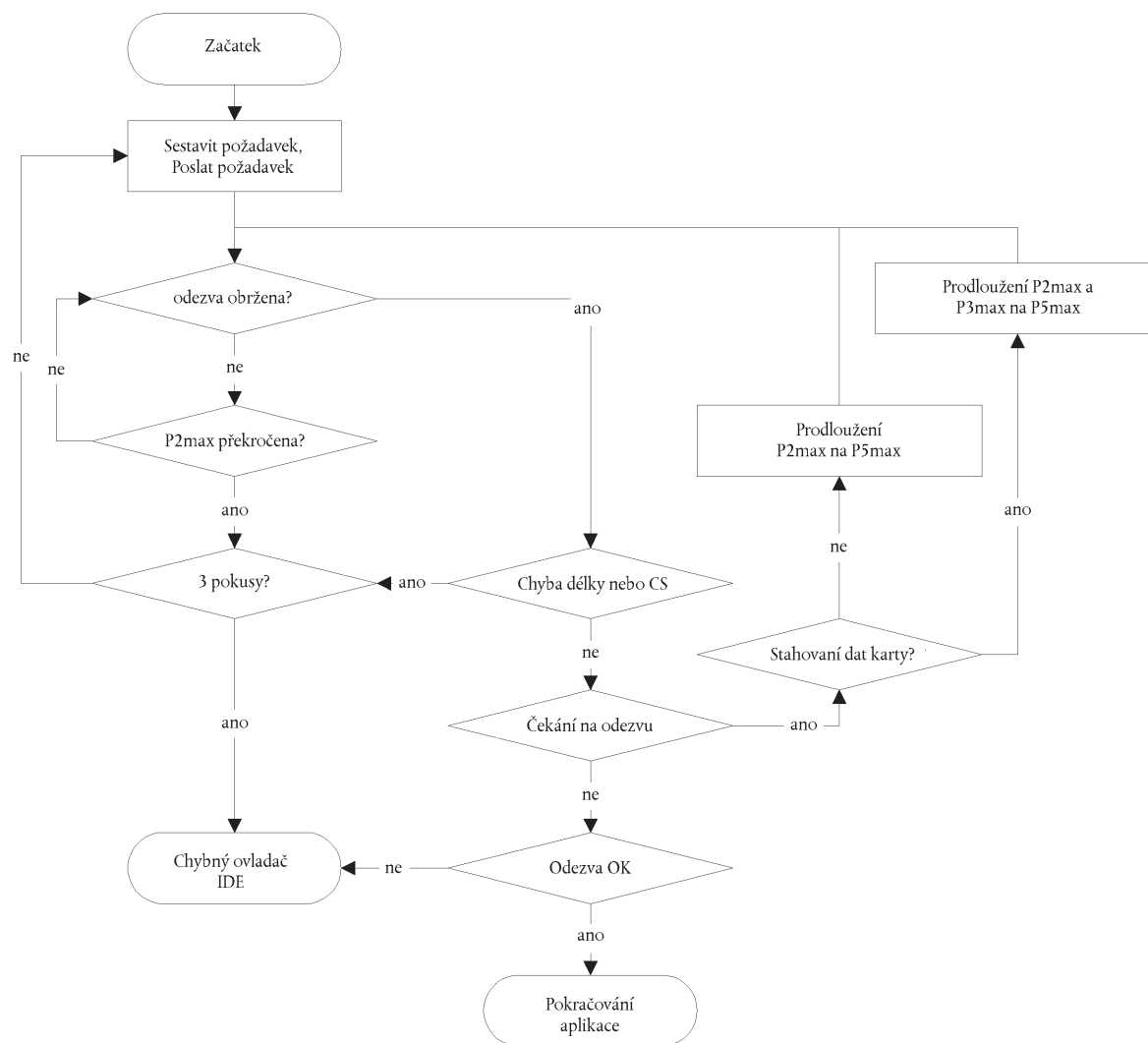
Obrázek 3 Zpracování chyb IDE
